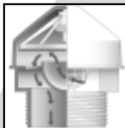
VALVE OPEN VÁLVULA ABIERTA SOUPAPE OUVERTE
